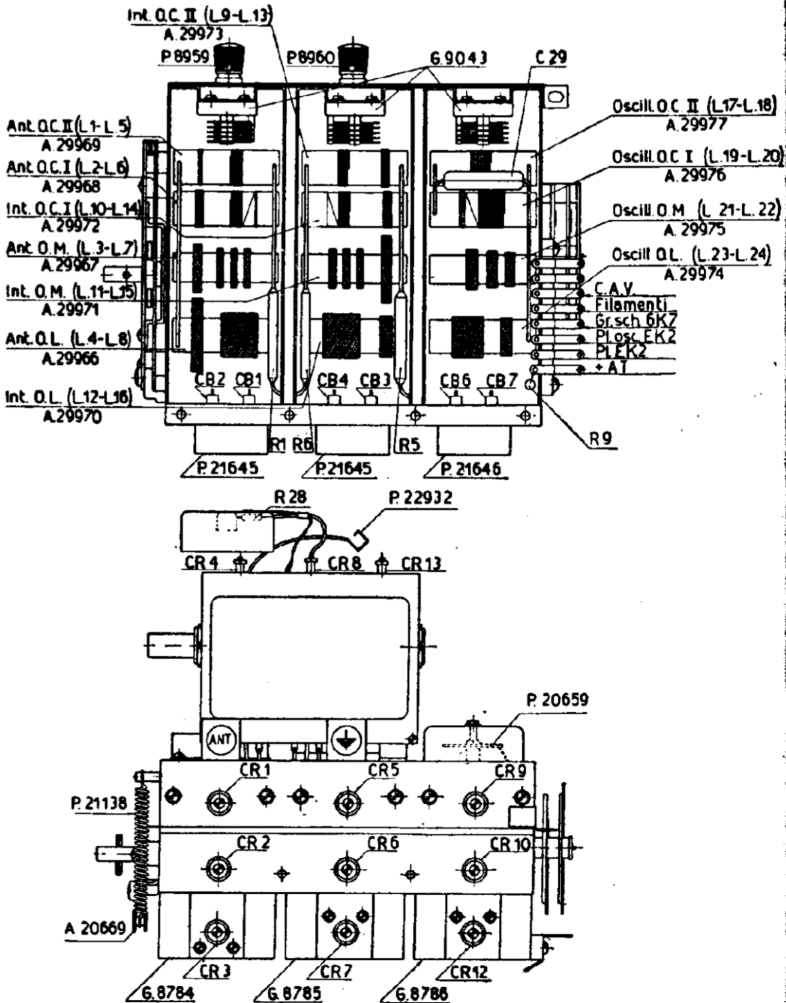
SAFAR. - Mod. 542. Castello di alta frequenza.
